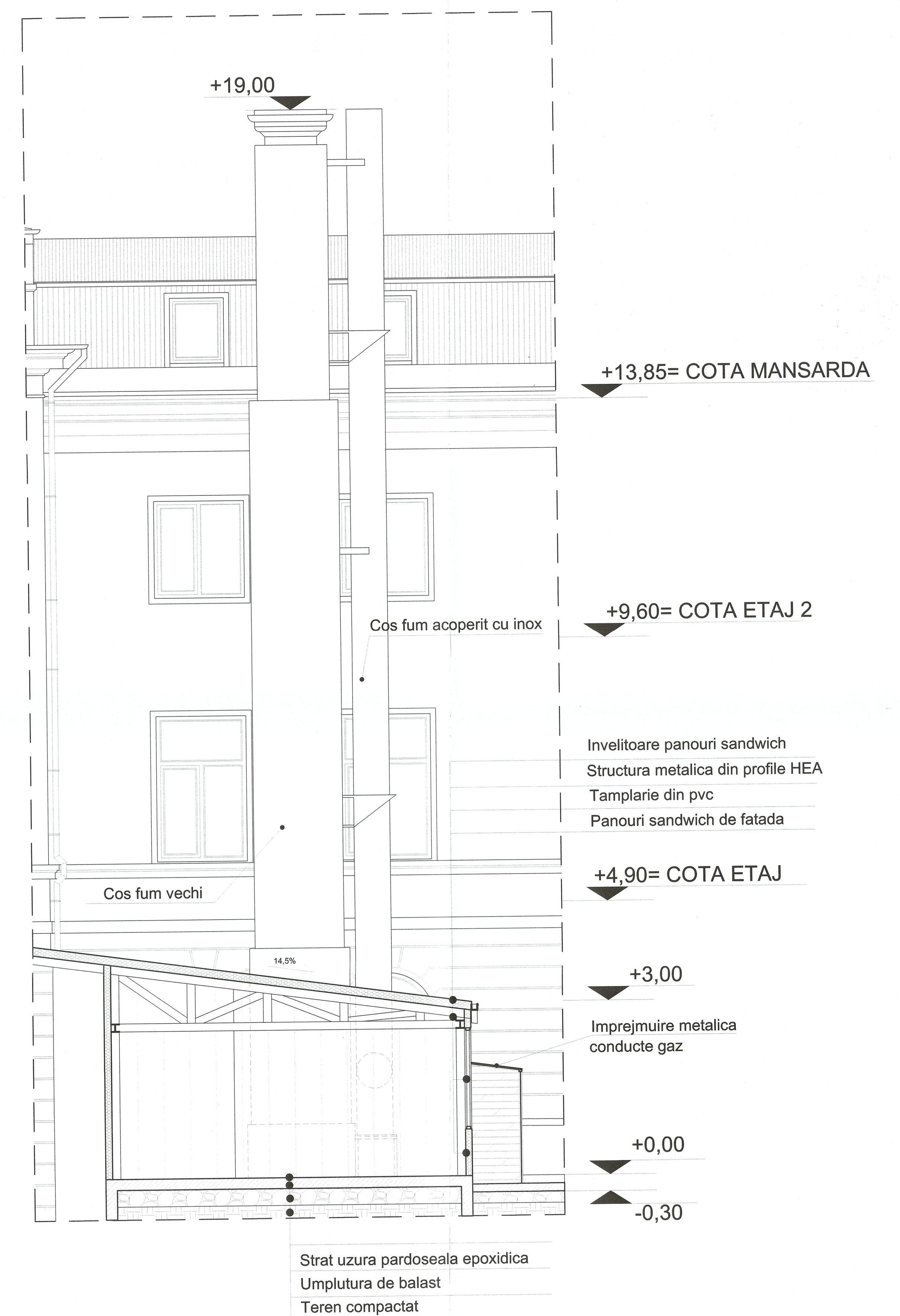
SECTIUNE CENTRALA TERMICA SI COS FUM
