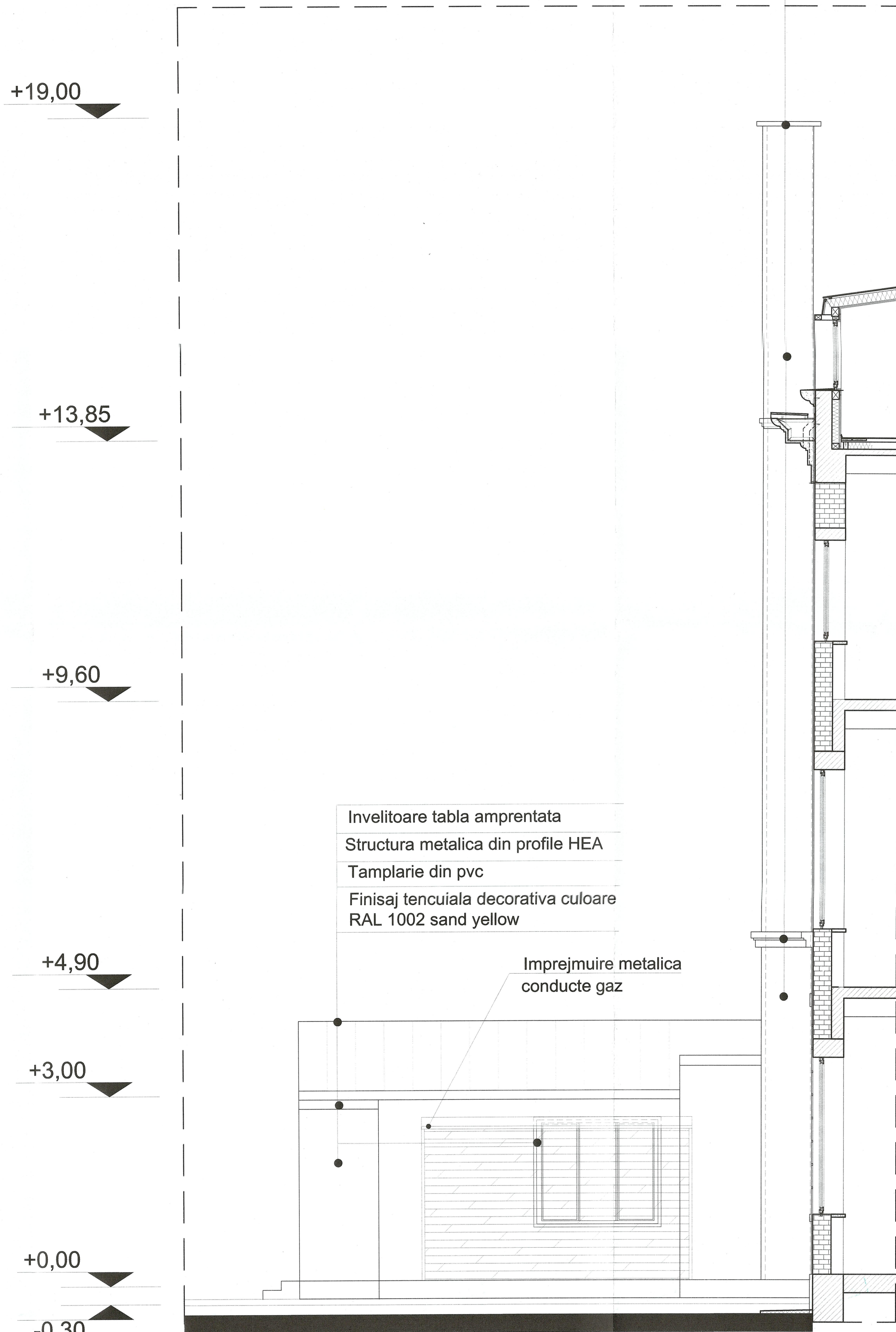
VEDERE LATERALA CENTRALA TERMICA SI COS DE FUM
